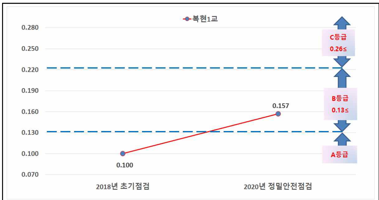
[그림 12.4.1] 복현1교 상태평가 결과 비교 그래프
