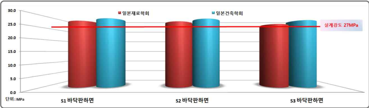
[그림 12.3.3] 반발경도법에 의한 비파괴강도 측정 결과-상부구조(바닥판하면)
