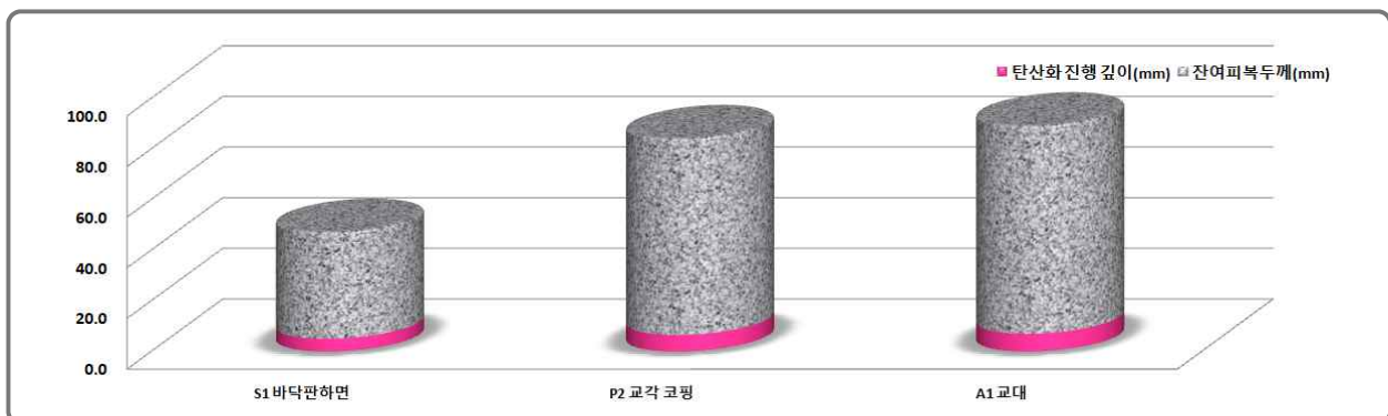
[그림 12.3.5] 탄산화깊이 및 잔여피복두께 측정결과
