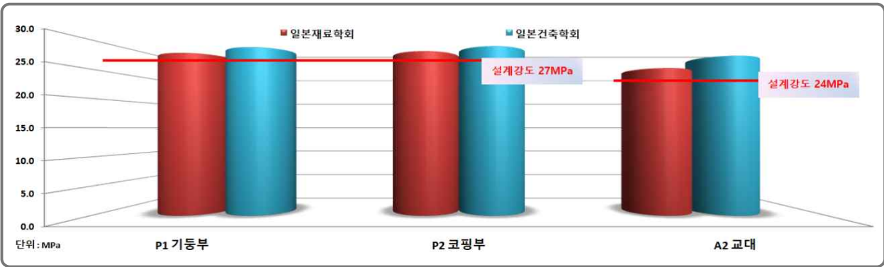
[그림 12.3.4] 반발경도법에 의한 비파괴강도 측정 결과-하부구조
